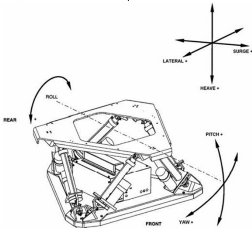
Fig. 1. Grados de Libertad de la plataforma definidos por el fabricante: yaw-pitch-roll-heave-sway-surge (guiñada-cabecceo-alabeo-elevación-abatimiento-avance) [10], [11].
